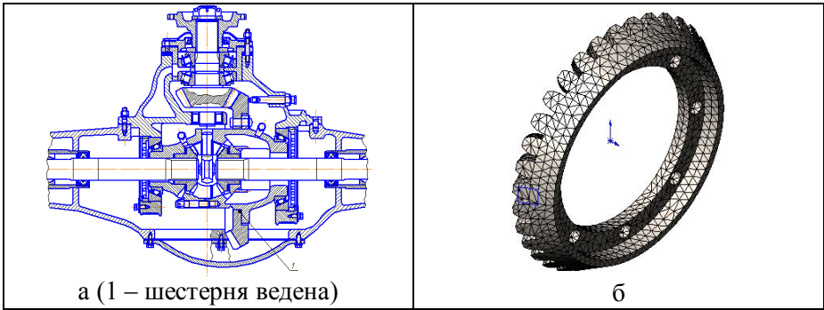
Рис. 1 – Креслення заднього моста автомобіля МАЗ-509 (а) і скінченно-елементна сітка моделі шестерні веденої (б)
