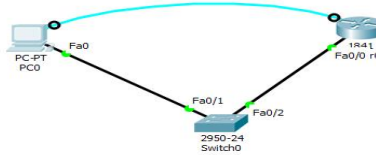
Рис. 1. Схема підключення
