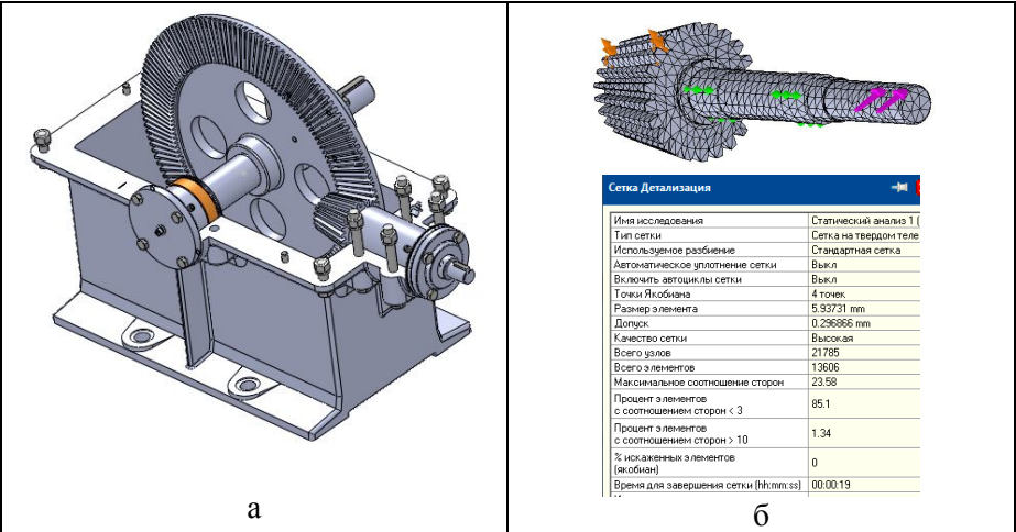
Рис. 1 – Твердотельная модель редуктора (а) та скінченно-елементна сітка моделі вал-шестерні з її параметрами (б)
